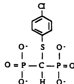
Tiludronate
